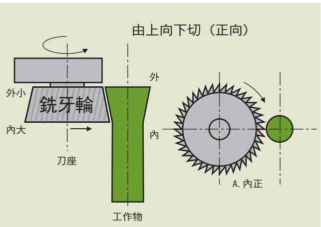
錐度螺紋之銑牙輪應用方向實例
